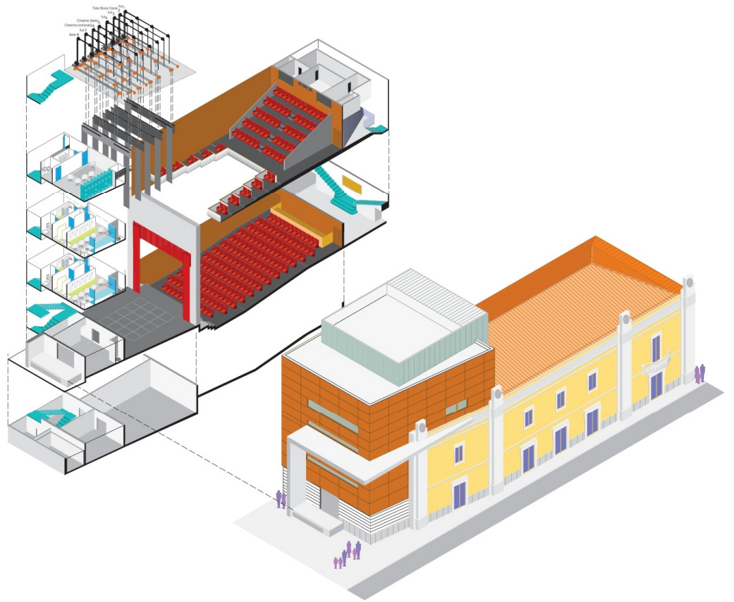
Casa da Cultura – Teatro Stephens Corte esquemático
